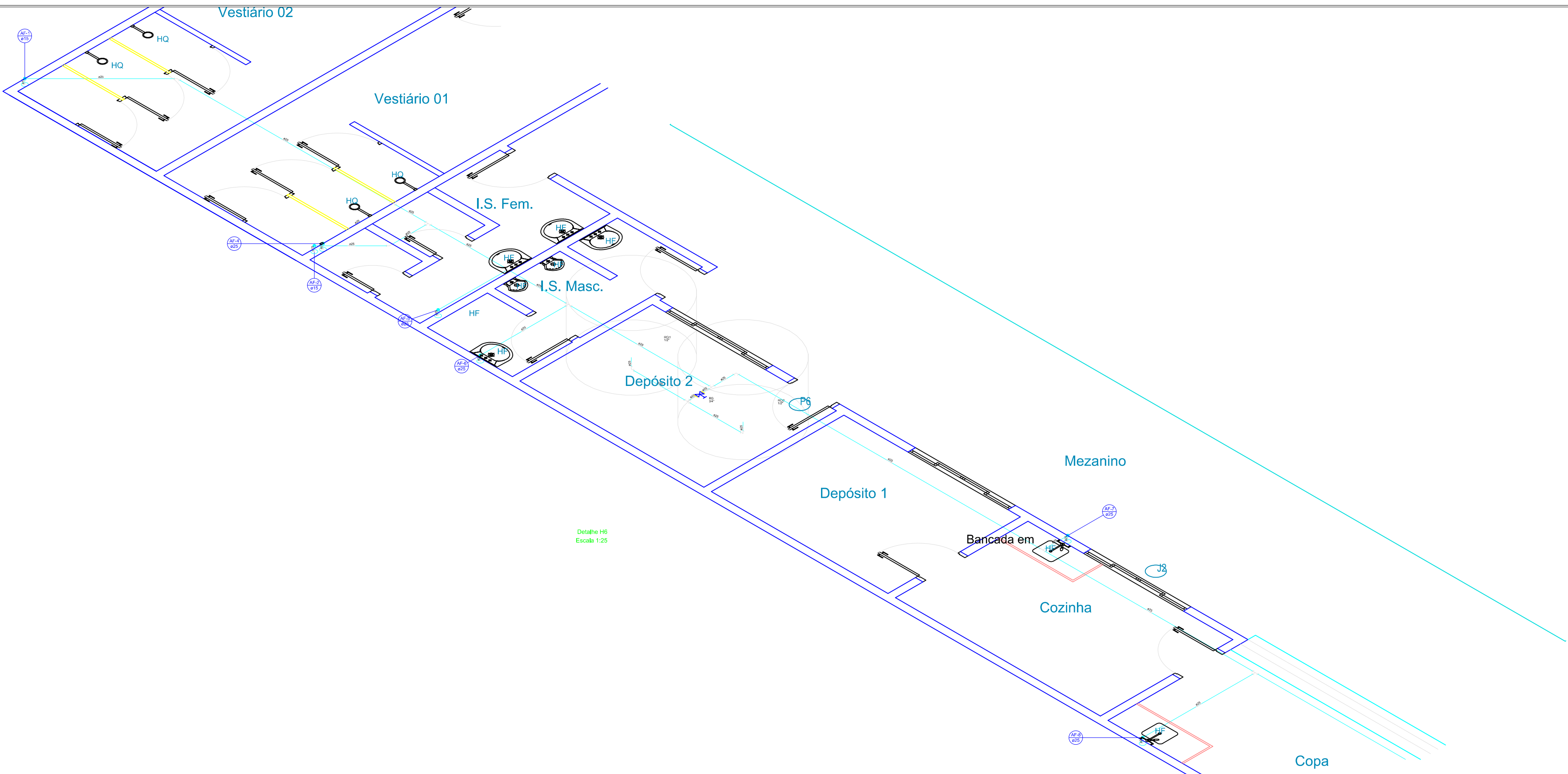
COBERTURA - HIDRÁULICO - PLANTA BAIXA Escala 1:100
